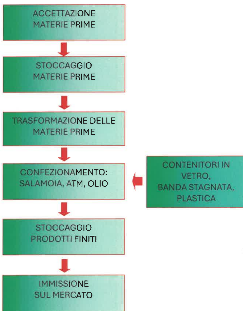
Figura 1 - Diagramma di flusso del processo produttivo:
